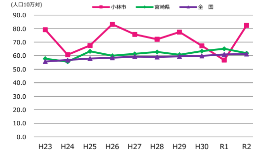
◆ 肺がん死亡率 年次推移 ◆
