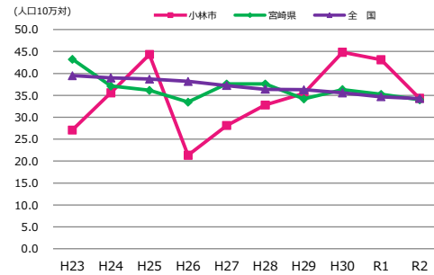
◆ 胃がん死亡率 年次推移 ◆
