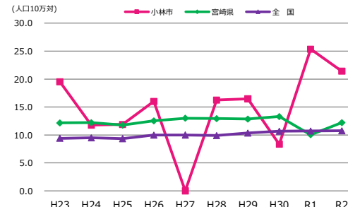
◆ 子宮がん死亡率 年次推移 ◆
