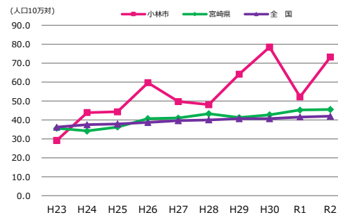
◆ 大腸がん死亡率 年次推移 ◆
