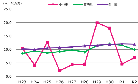
◆ 乳がん死亡率 年次推移 ◆
